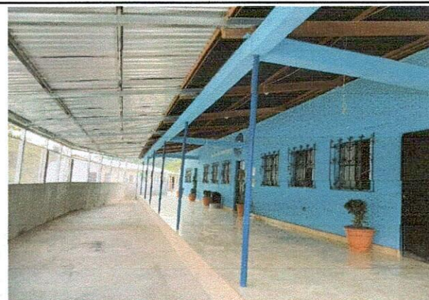
Foto 4: Instalacion de estructura de techo y cubierta de lamina calibre 26 de una caida de agua para patio.
